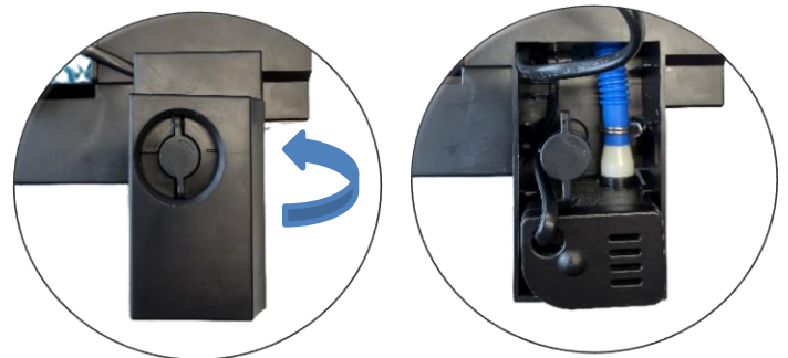
Abb. 4.7.2 Abdeckung der Wasserpumpe (links: geschlossen; rechts: geöffnet)
