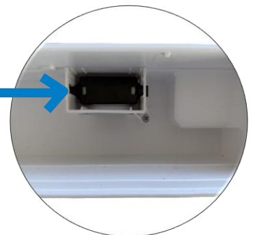
Abb. 4.6.1 Schwimmer
